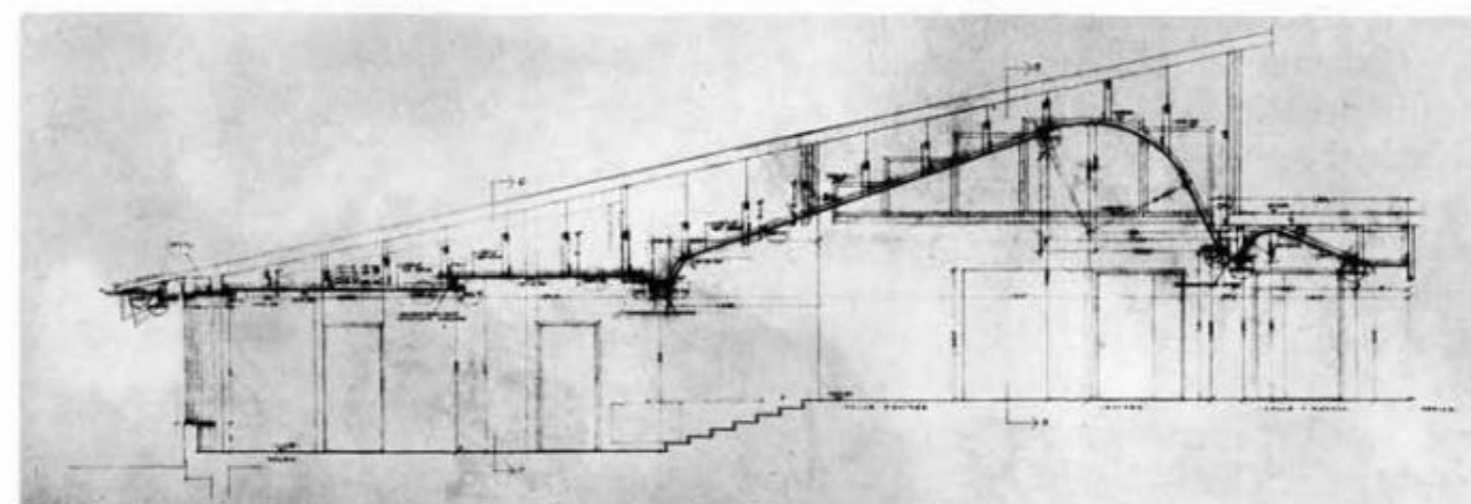
153. Aalto, Maison Carré, Bazoches. Section
